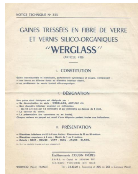
Notice technique d'une gaine en fibre de verre et vernis silico-organiques fabriquée chez Cousin à Wervicq-Sud (MRc2561).
